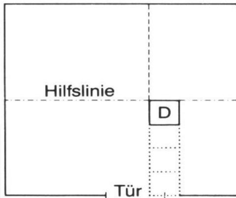
Anordnung der erste Fliesenreihe
